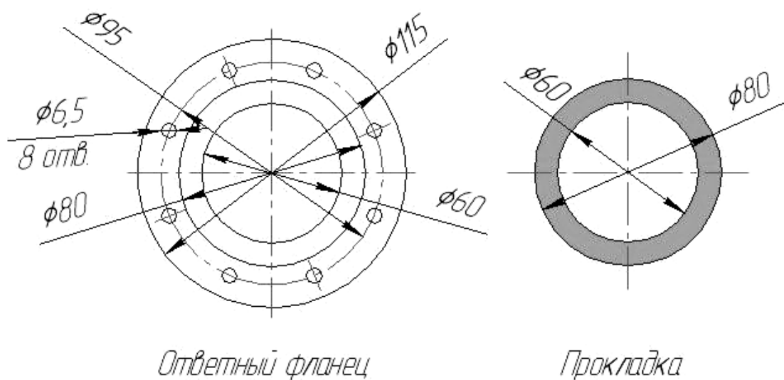
Рис.5. Габаритные размеры установочного фланца и прокладки для сигнализаторов
